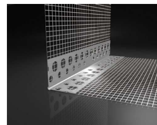
Angolare ALLUMINIO RETE 8X12 CM.
